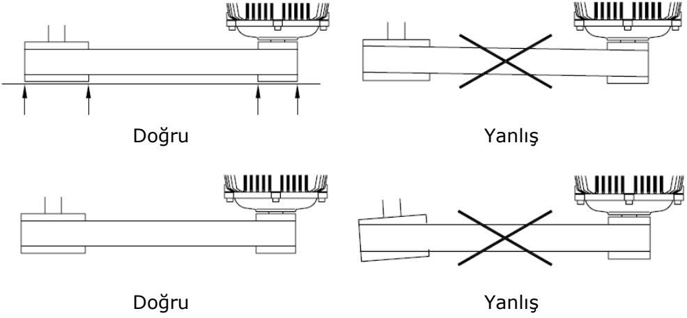
Şekil-2: Kayış ve kasnak hizalaması
