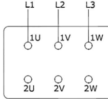
Şekil-3: Doğrudan yol verme şeması
