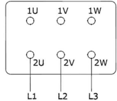
Şekil-4: Çift hızlı motorlar için bağlantı şemaları
