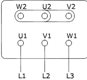
Şekil-3: Doğrudan yol verme şeması
